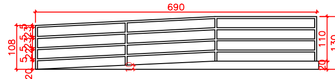
Rampa de Acesso ESC-1/50
