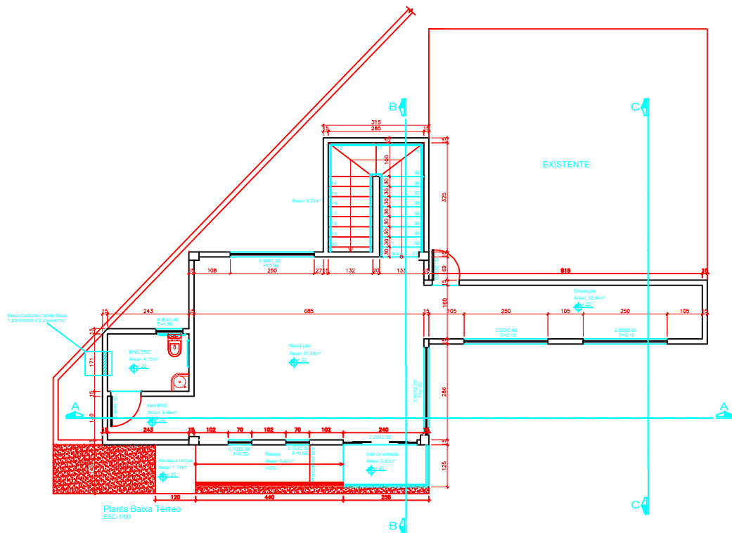
Planta Baixa 1º Piso ESC-1/50
