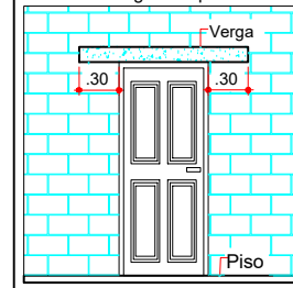
Detalhe - vergas em portas
