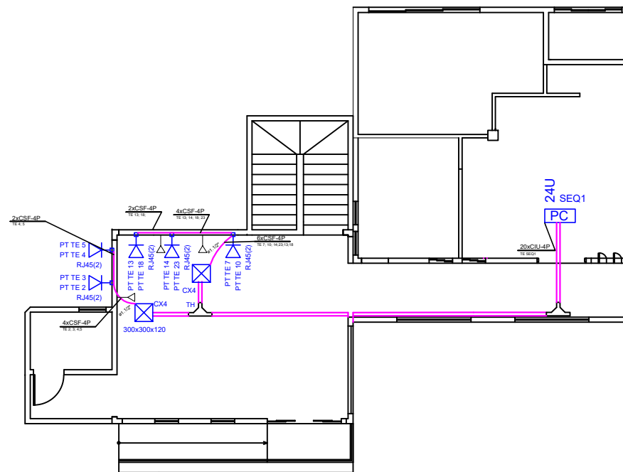
PLANTA BAIXA DE LÓGICA ESCALA: 1/100
