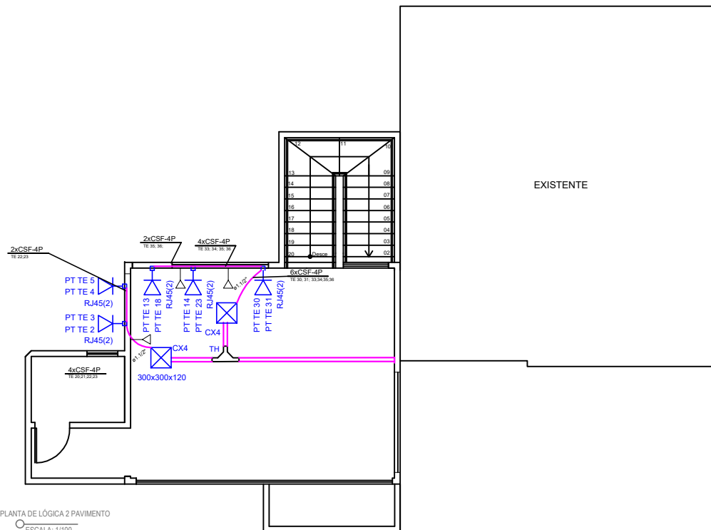
PLANTA BAIXA DE LÓGICA ESCALA: 1/100
